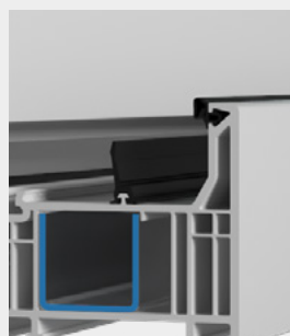
Středové těsnění
